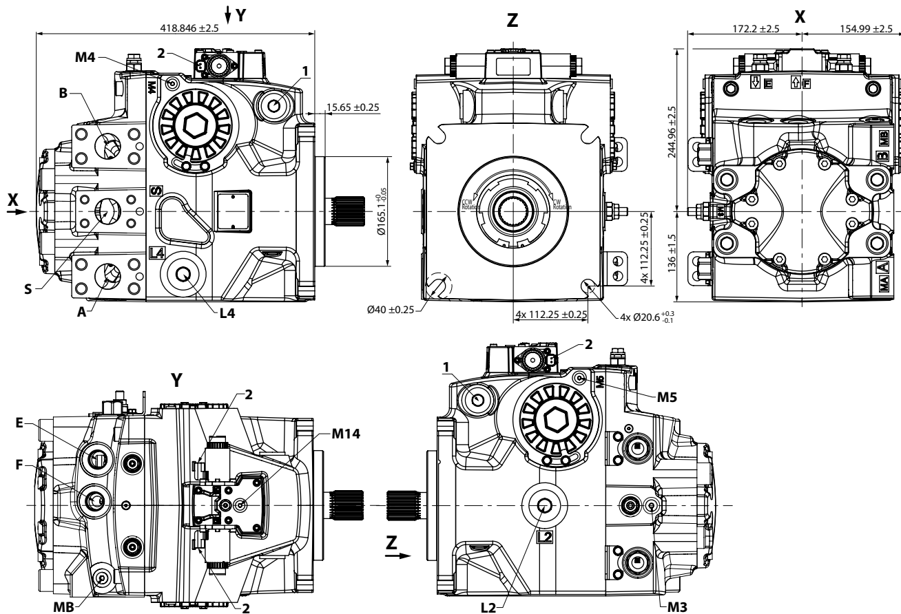
Ports per ISO 11 926-1
