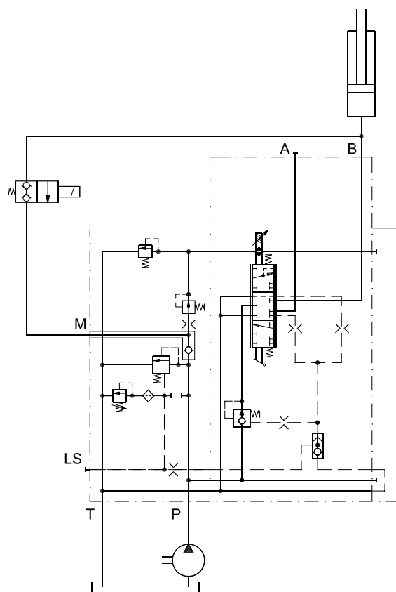
Гидравлическая схема
