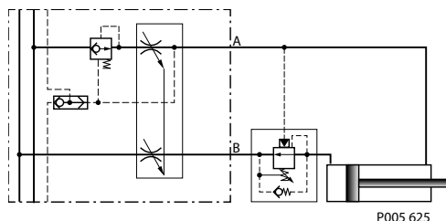
Рис. 4. Золотник управления расходом, не зависящий от давления (золотник FC)
