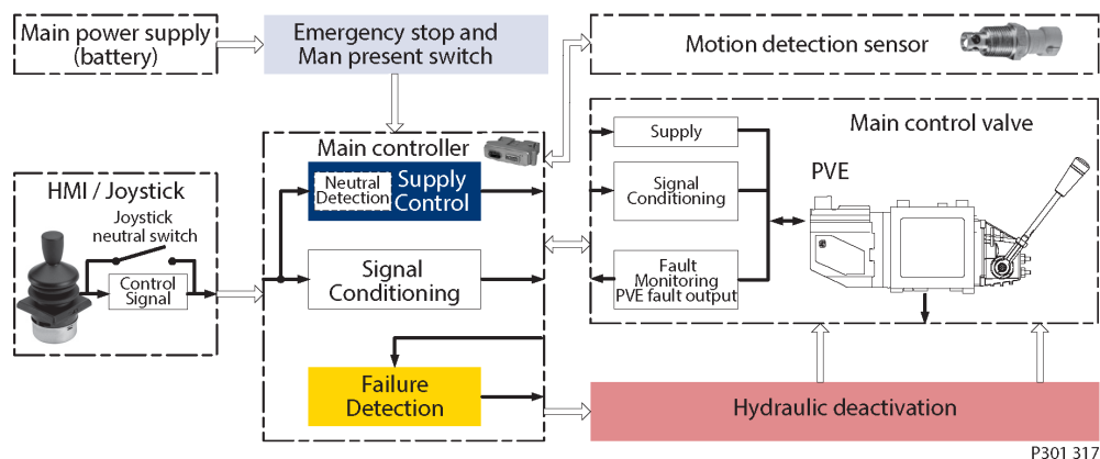
Блок-схема электрооборудования для приведенного выше рисунка
