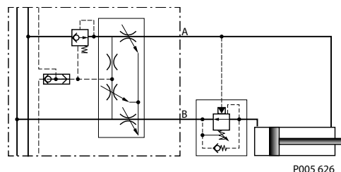
Рис. 5. Золотник управления расходом, зависящий от давления (золотник PC)
