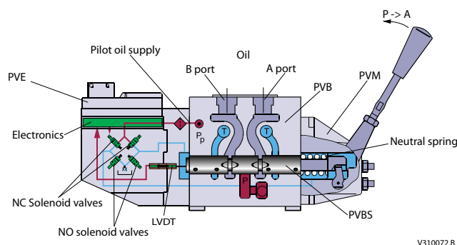
Секция распределителя с обозначениями — стандартное исполнение — вид со стороны PVP
