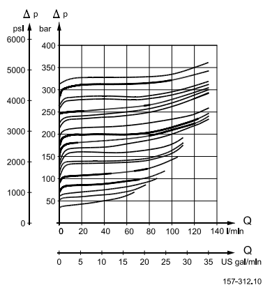
PVLP, характеристика ударного клапана
