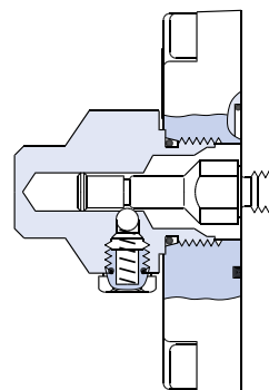
PVMR, фрикционный стопор
