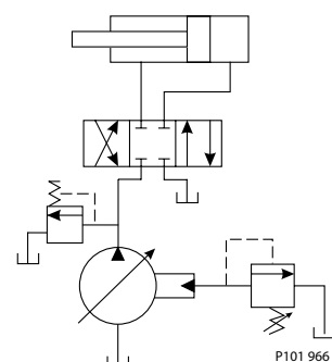
Контур с закрытым центром и РС-регулятором с дистанционным управлением
