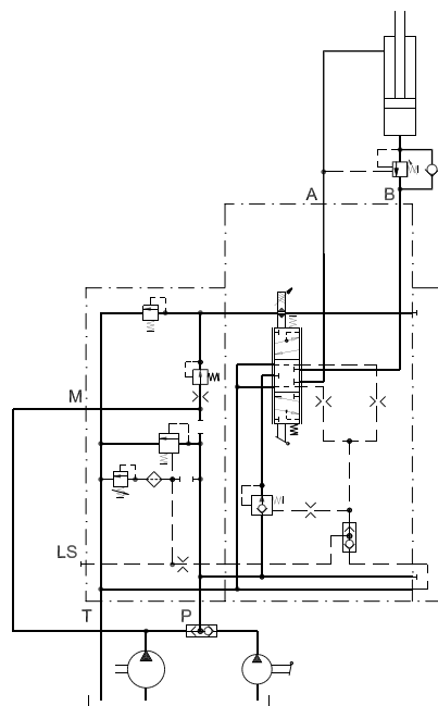
Гидравлическая схема
