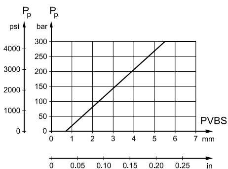
Зависимость давления насоса от перемещения золотника
