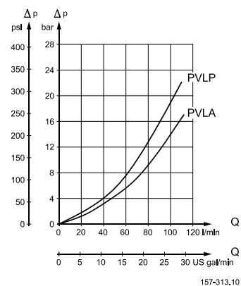
PVLA, характеристика антикавитационного клапана
