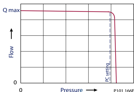
Рабочая характеристика
