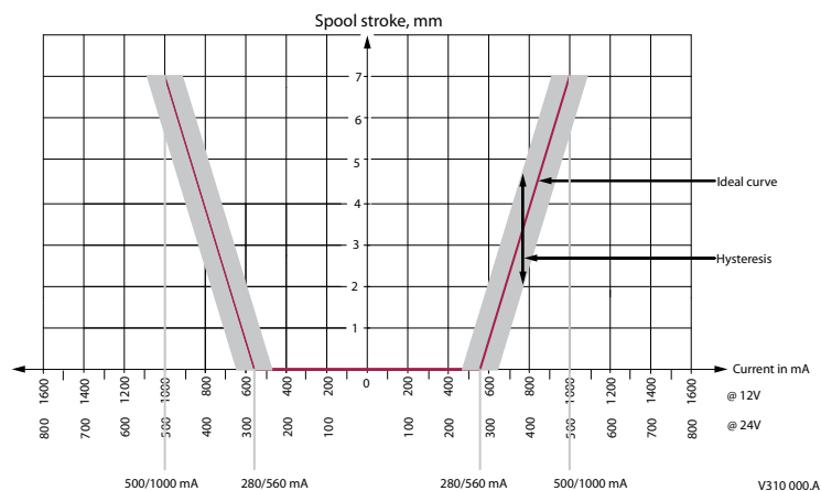
Характеристика PVHC — зависимость перемещения золотника от тока
