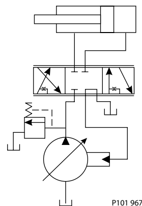
Гидросхема LS-регулирования
