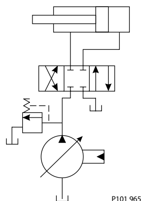
Простая система с закрытым центром
