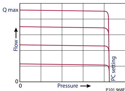
Рабочая характеристика
